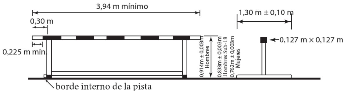
Figura (a) RT23 - Ejemplo de una valla de obstáculos
