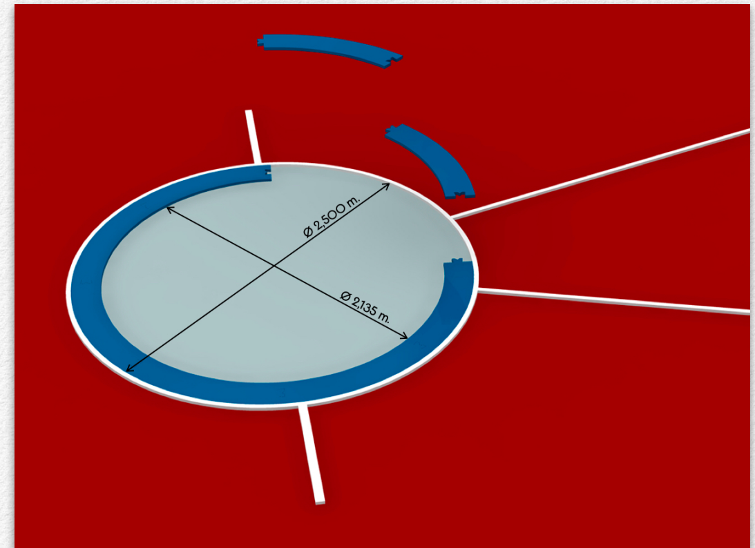
Círculo de Lanzamiento de Disco con reductor para Lanzamiento Martillo. Mondo.
