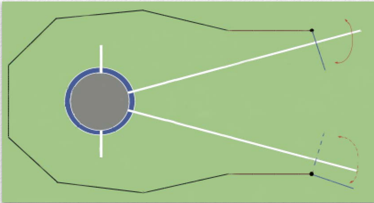
Jaula para Lanzamiento de Disco y Martillo, disposición para Lanzamiento de Martillo con utilización de reductor.
