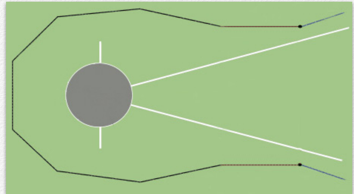
Jaula para Lanzamiento de Disco y Martillo, disposición para Lanzamiento de Disco.
