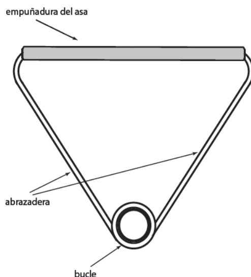
Figura (b) RT36 - Empuñadura de martillo genérica
