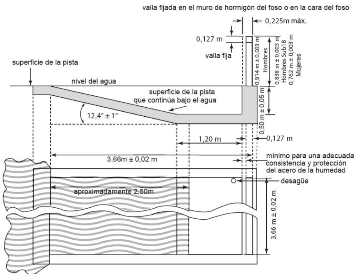
Figura (b) RT23 - Ría
