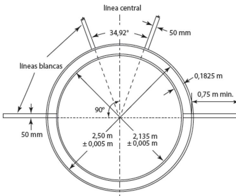
Figura (d) RT32 - Disposición de círculos concéntricos para Lanzamientos de Disco y Martillo
