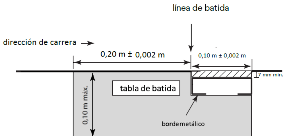
Figura (a1) RT29- Tabla de batida con tabla ciega
