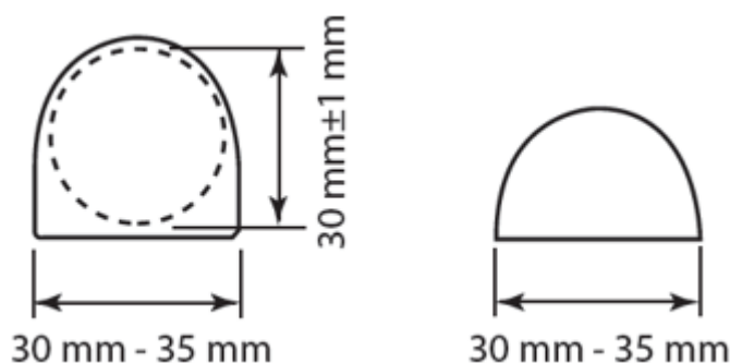
Figura RT26.- Extremos alternativos para el listón
