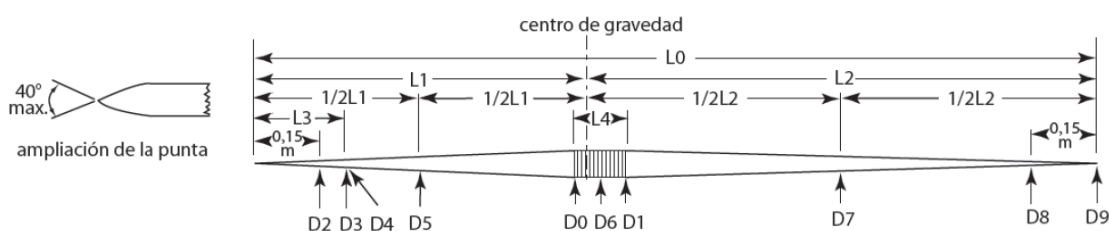
Figura RT38 - Jabalina Internacional
